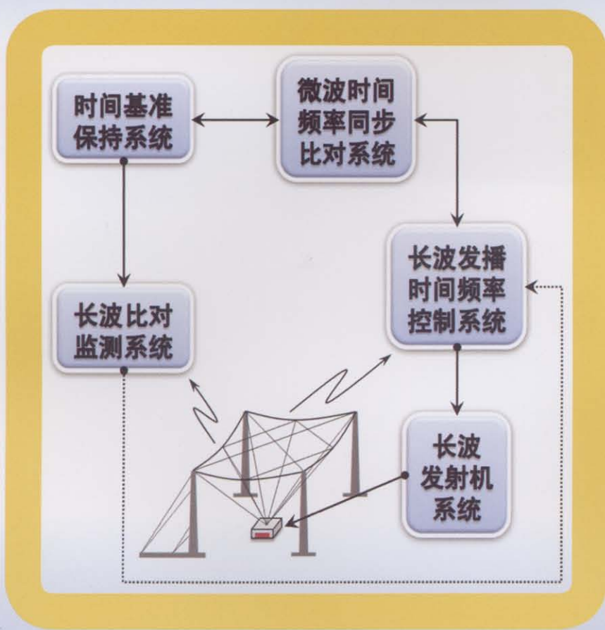
发射机控制及信号监测系统
